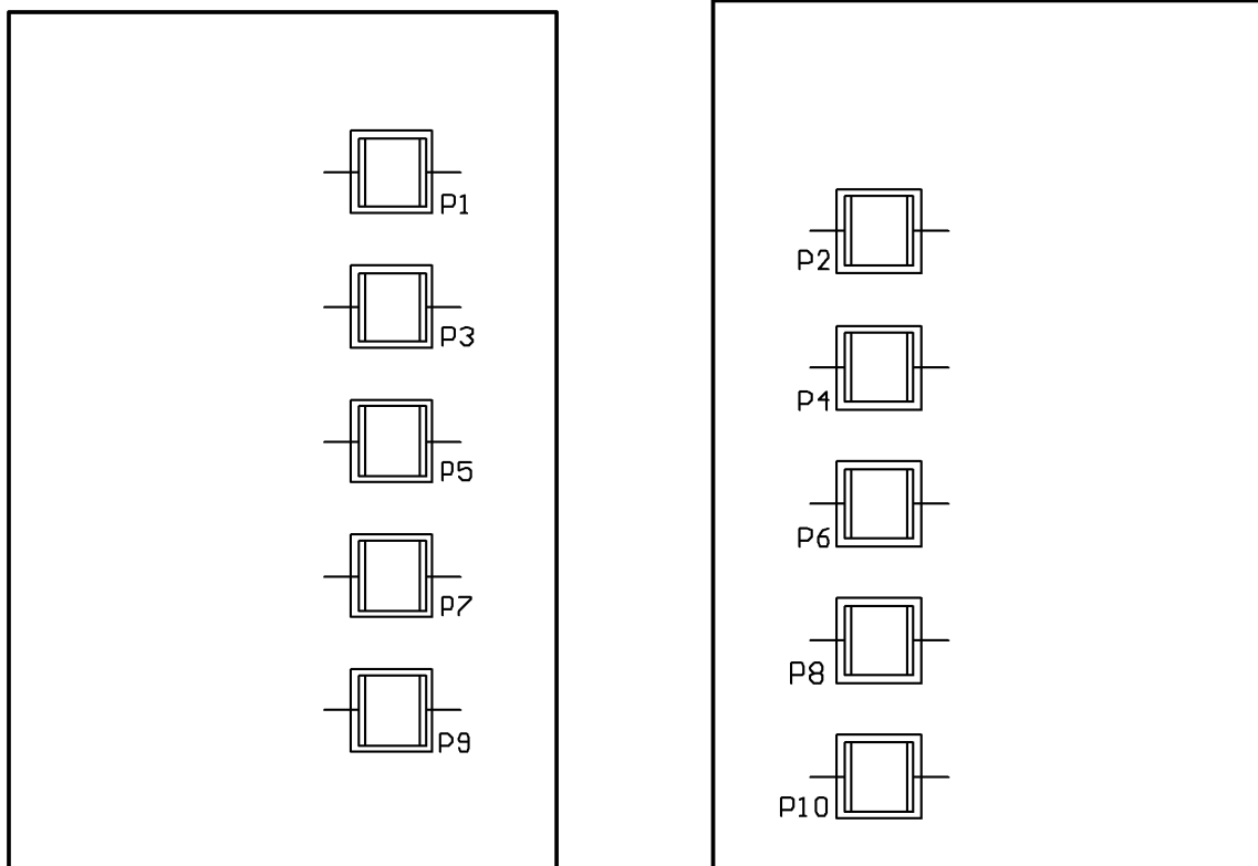
Сборочный чертеж платы кабеля электродного МТЦ.30.03.501СБ (сторона 1 и 2)
