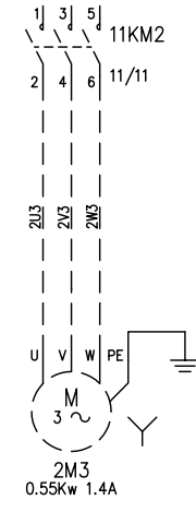
POMPA CESTI OPZIONALE BASKETS PUMP OPTIONAL
