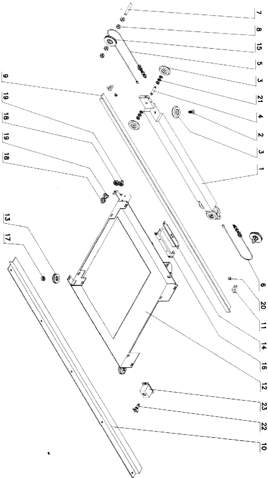
Чертеж E2608_Изм.02
