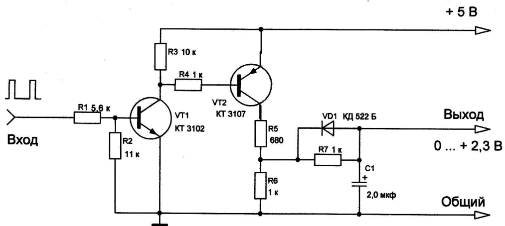
Преобразователь ШИМ 10 кГц в аналоговое напряжение 0..2,3 В
