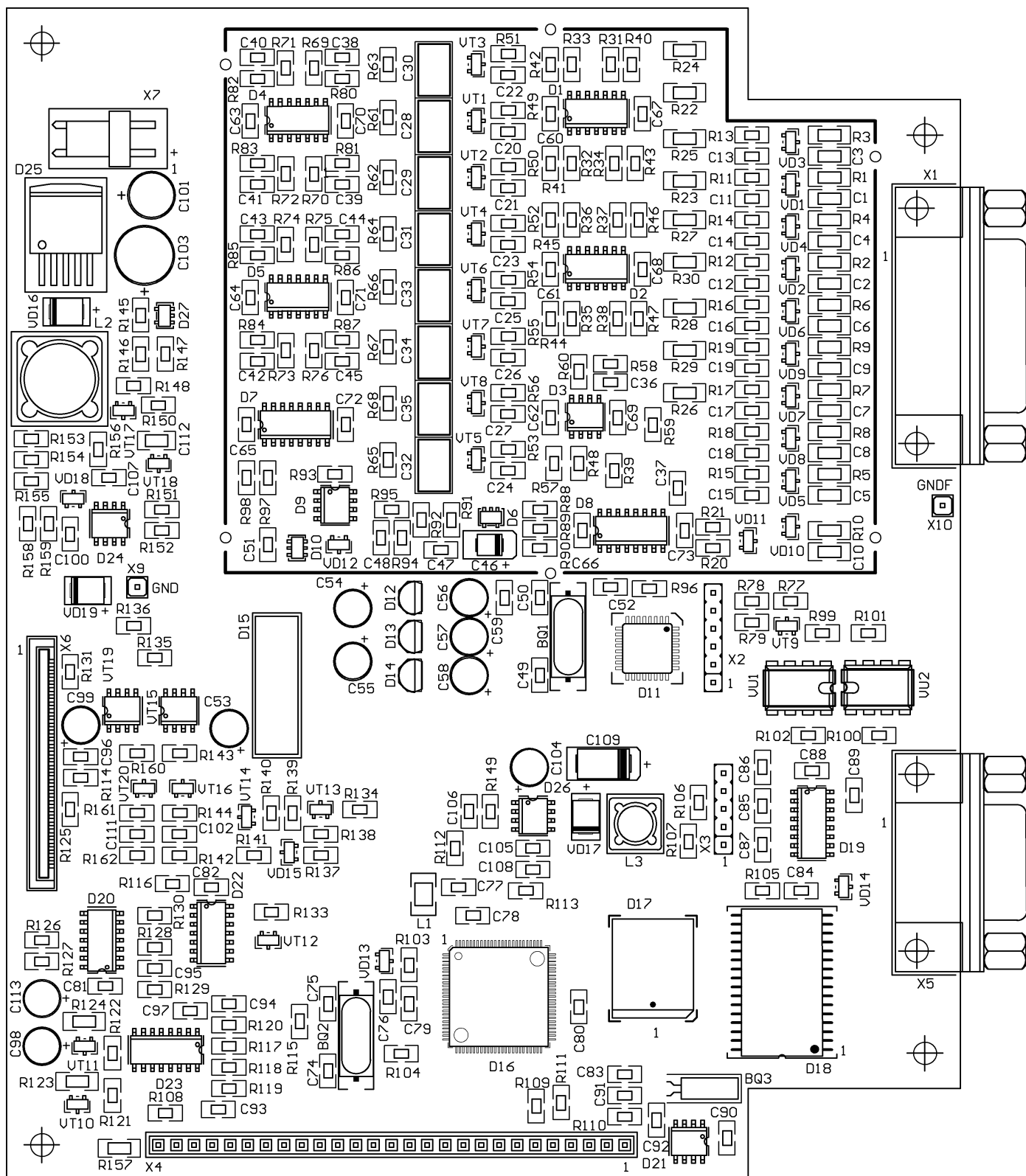
Сборочный чертеж модуля ЭКЗТ МТЦ.30.01.502СБ (сторона 1)
