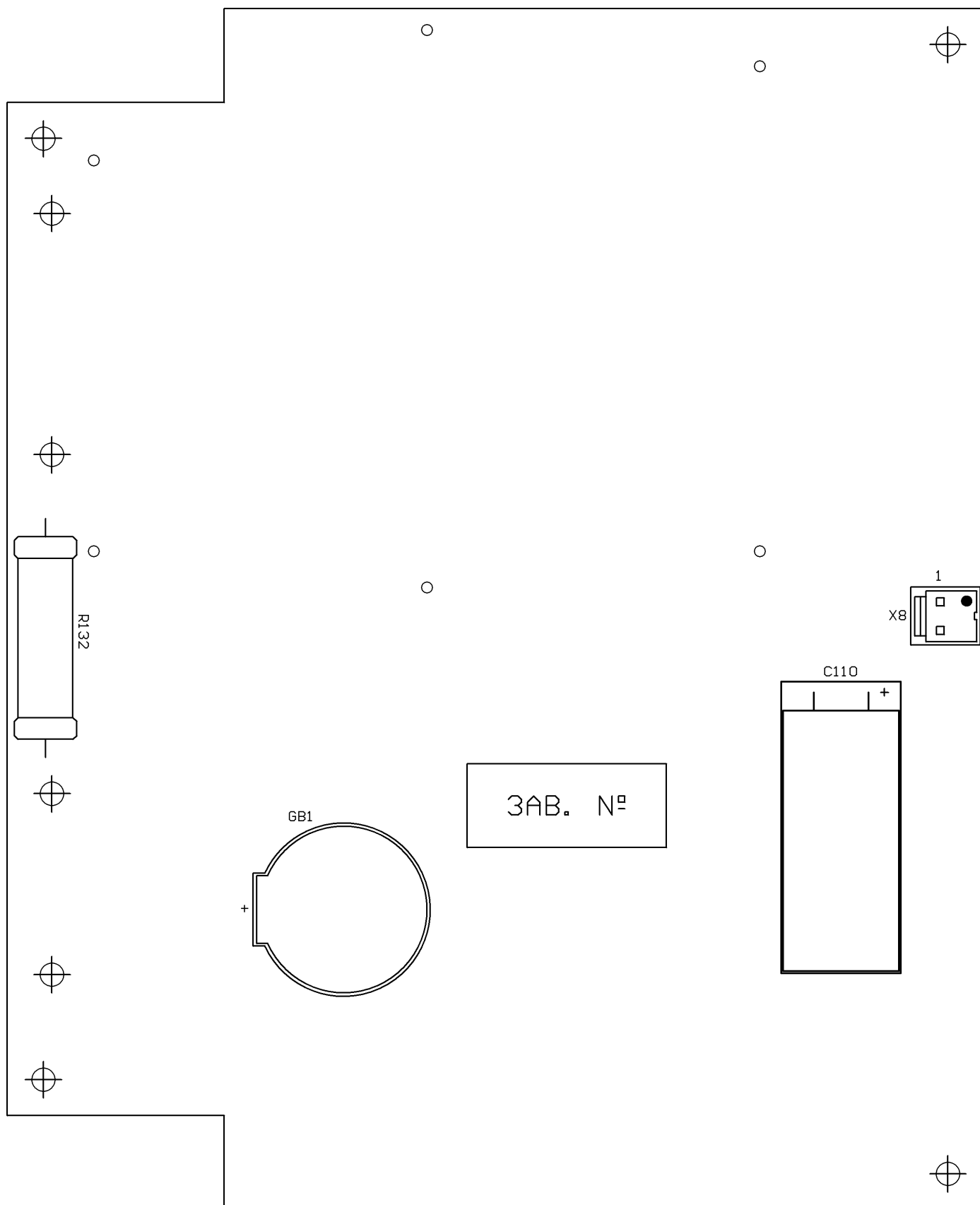
Сборочный чертеж модуля ЭКЗТ МТЦ.30.01.502СБ (сторона 2)
