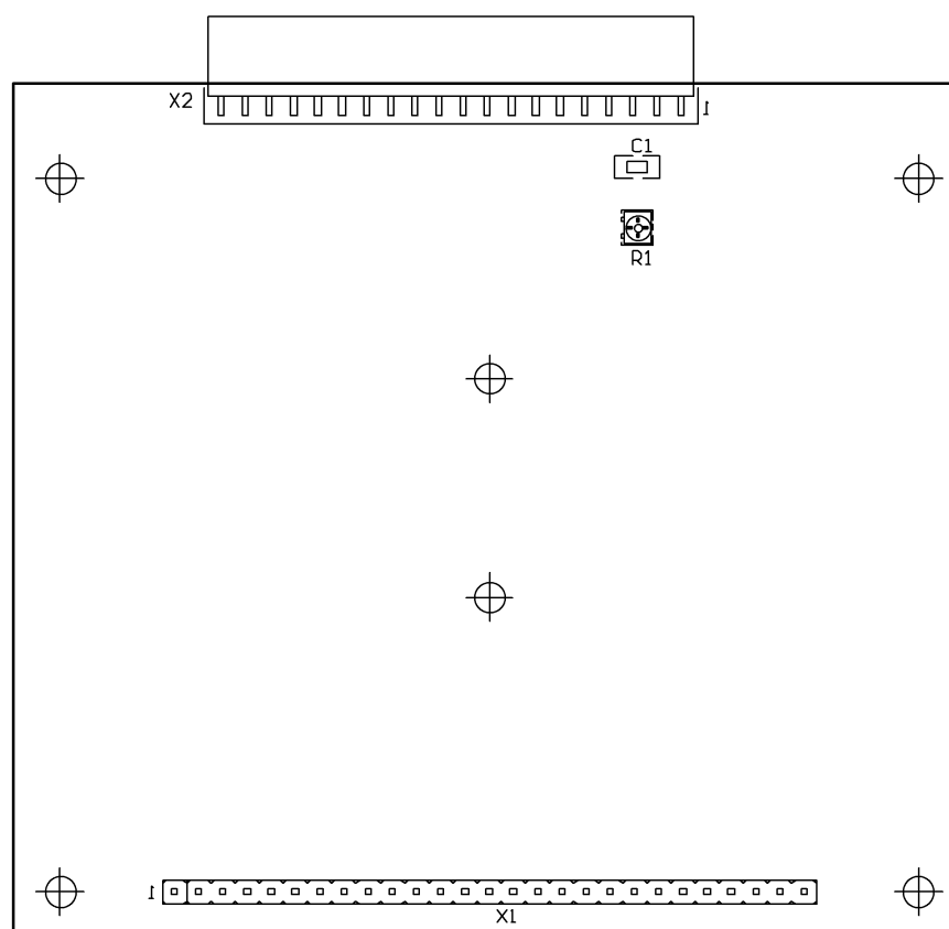
Сборочный чертеж платы клавиатуры МТЦ.30.02.502СБ (сторона 2)
