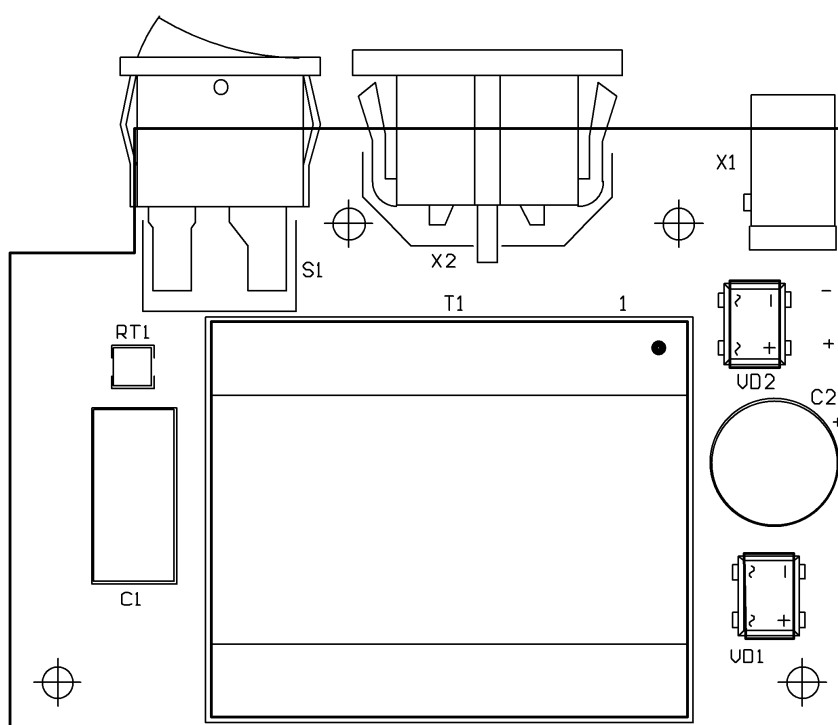
Сборочный чертеж платы узла питания МТЦ.30.04.502СБ
