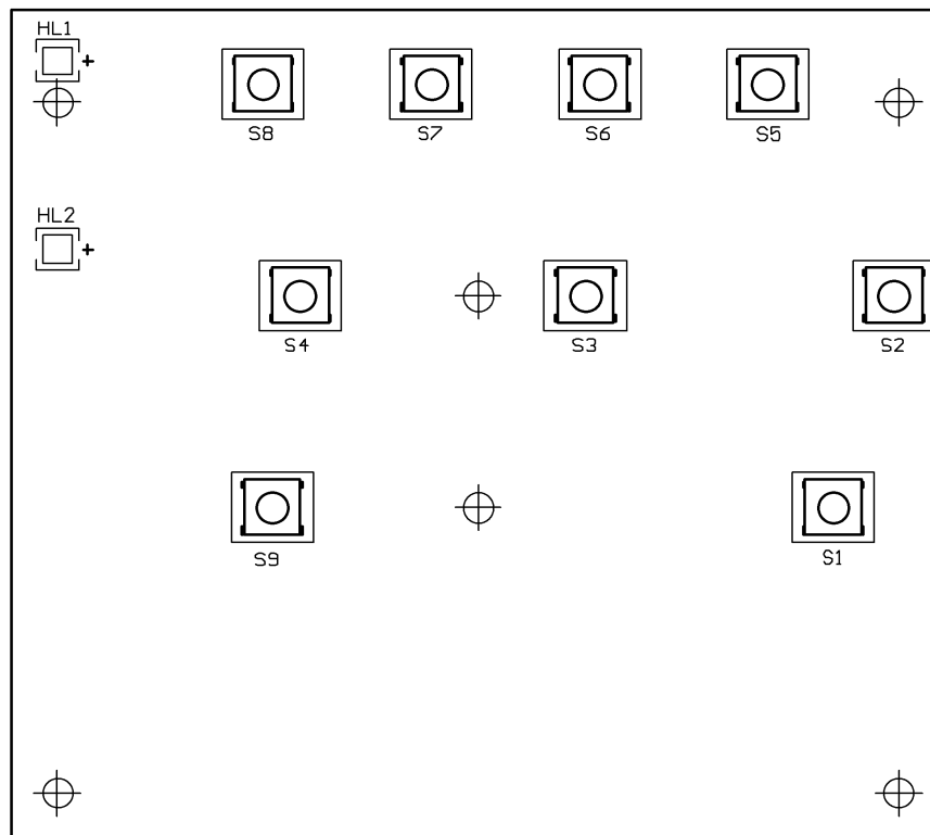
Сборочный чертеж платы клавиатуры МТЦ.30.02.502СБ (сторона 1)
