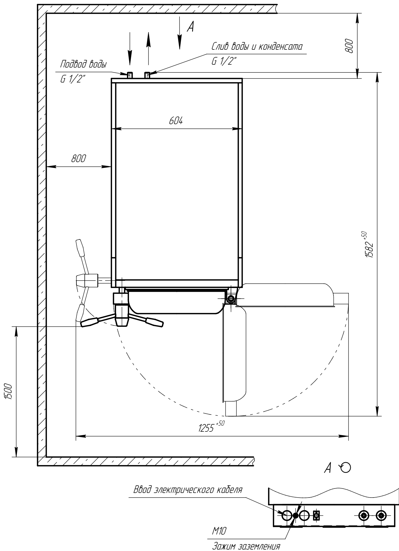
Рисунок 6 – Стерилизатор паровой ГК-100-3. Установочные размеры
